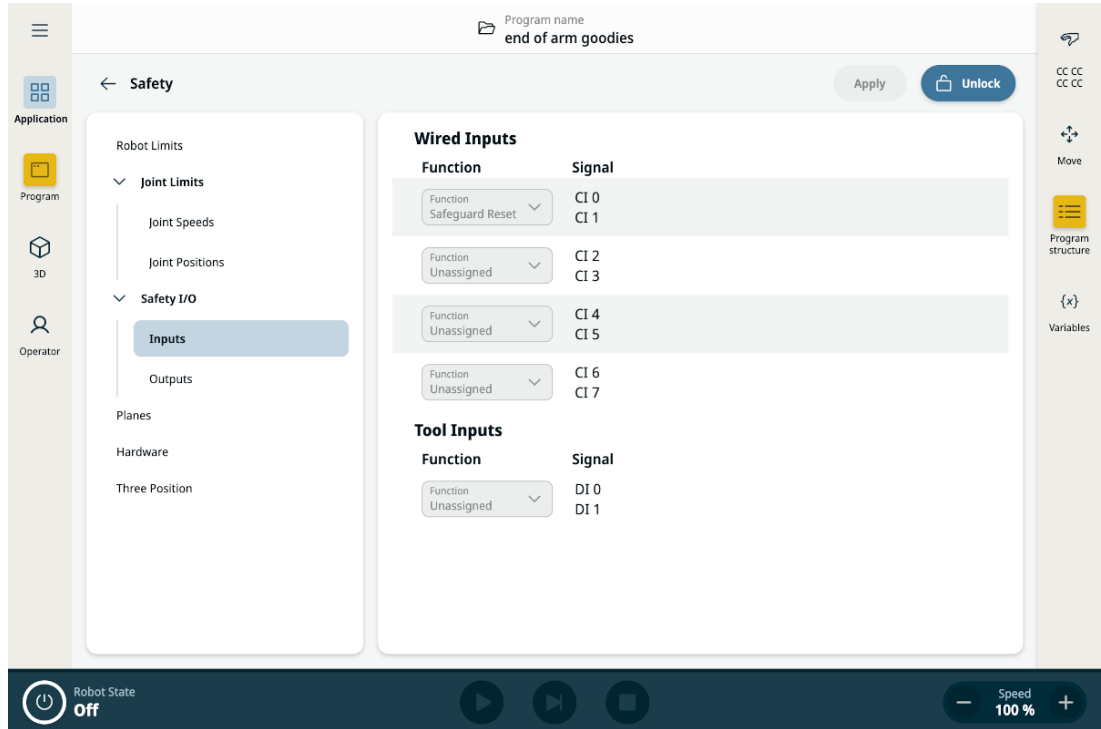
图 1.4: 显示输入信号的 PolyScope X 屏幕。
