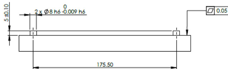
1.2: 机器人基座安装板
